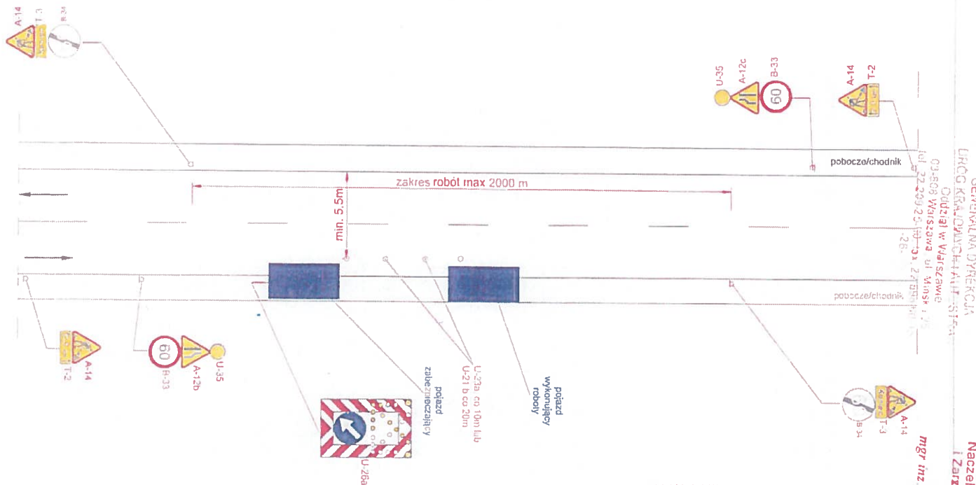
rys. 17 Roboty szybko postępujące, zajęcie pobocza/chodnika oraz części pasa ruchu
